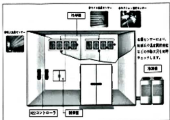
Fig. 1 TKSシステム設置図
