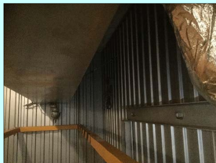
吸込み温度センサ取付
